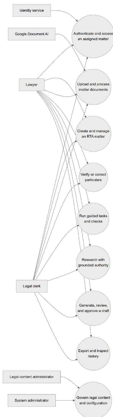
Figure 3. VO use-case diagram.
